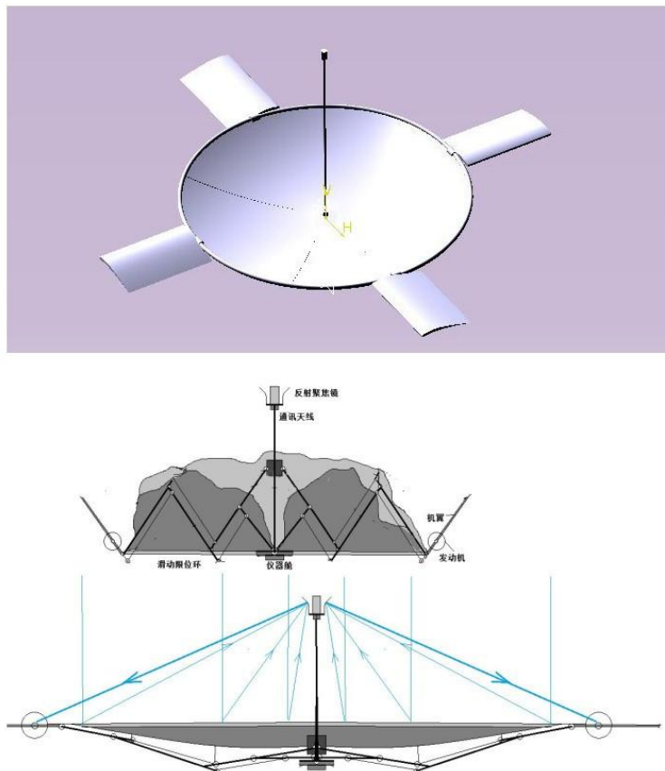
图为“夸父”号金星探测器设计图样
